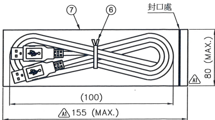
包裝示意圖
